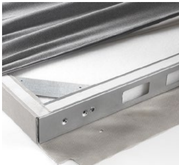
Cadre métallique perforé sur les 4 côtés
